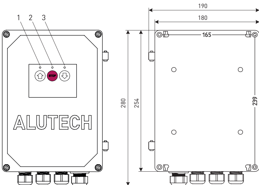
Рисунок 1. Блок управления (размеры указаны в миллиметрах)
