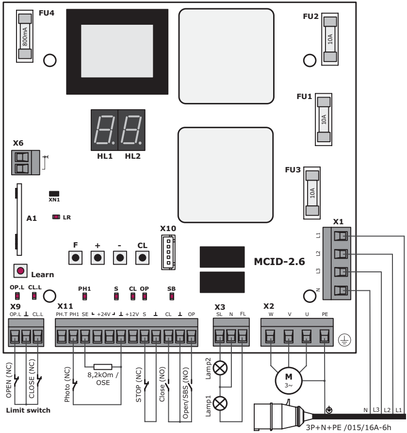
Малюнок 2. Електронний модуль блока керування
