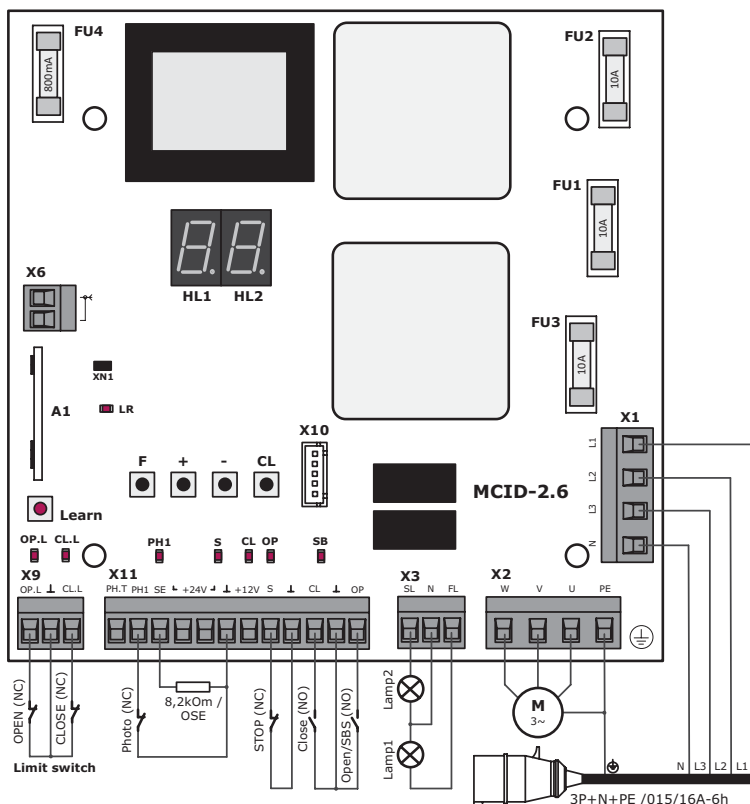
Рисунок 2. Электронный модуль блока управления
