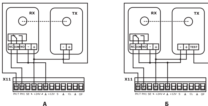
Малюнок 5. Підключення фотоелементів
