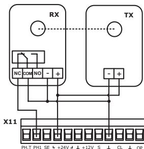
Малюнок 4. Підключення фотоелементів
