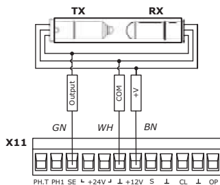
Рисунок 3. Подключение оптоэлектронного датчика безопасности нижней кромки полотна ворот/OSE (Optoelectronic Safety Edge)
