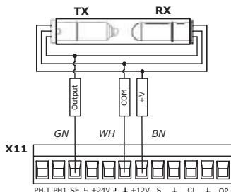
Малюнок 3. Підключення оптоелектронного датчика безпеки нижньої кромки полотна воріт/ OSE (Optoelectronic Safety Edge)
