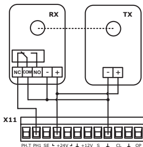
Рисунок 4. Подключение фотоэлементов
