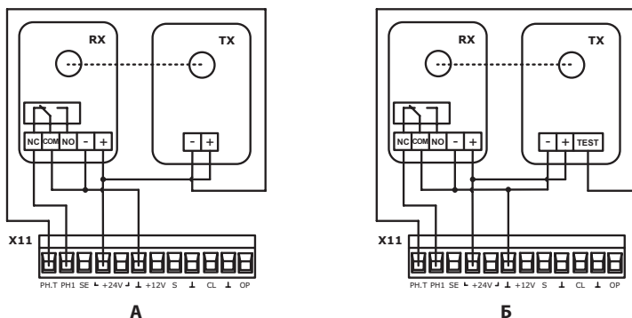
Рисунок 5. Подключение фотоэлементов
