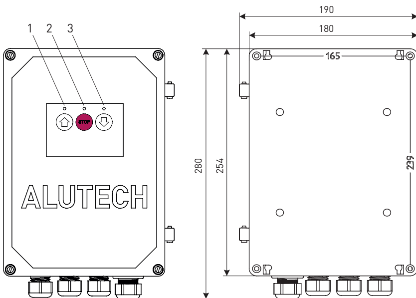
Малюнок 1. Блок керування (розміри вказані в міліметрах)
